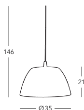
0051.31.6 Hängeleuchte / hanging lamp 1 Ip., E27, 60 W
